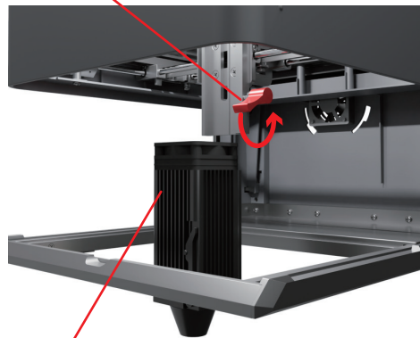
Laser Module
